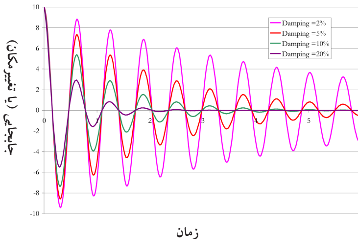
شکل ۲-۱ اثر میرایی بر کاهش پاسخ سازه
