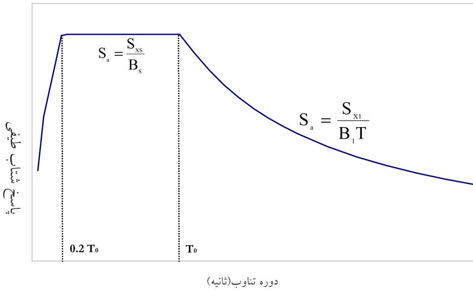
شکل ۴-۲ طیف FEMA
