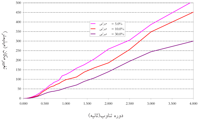
شکل ۴-۲ طیف FEMA
